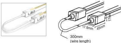
CONECTOR RECTO DE PUENTE JUMPER CONNECTOR-STRAIGHT
